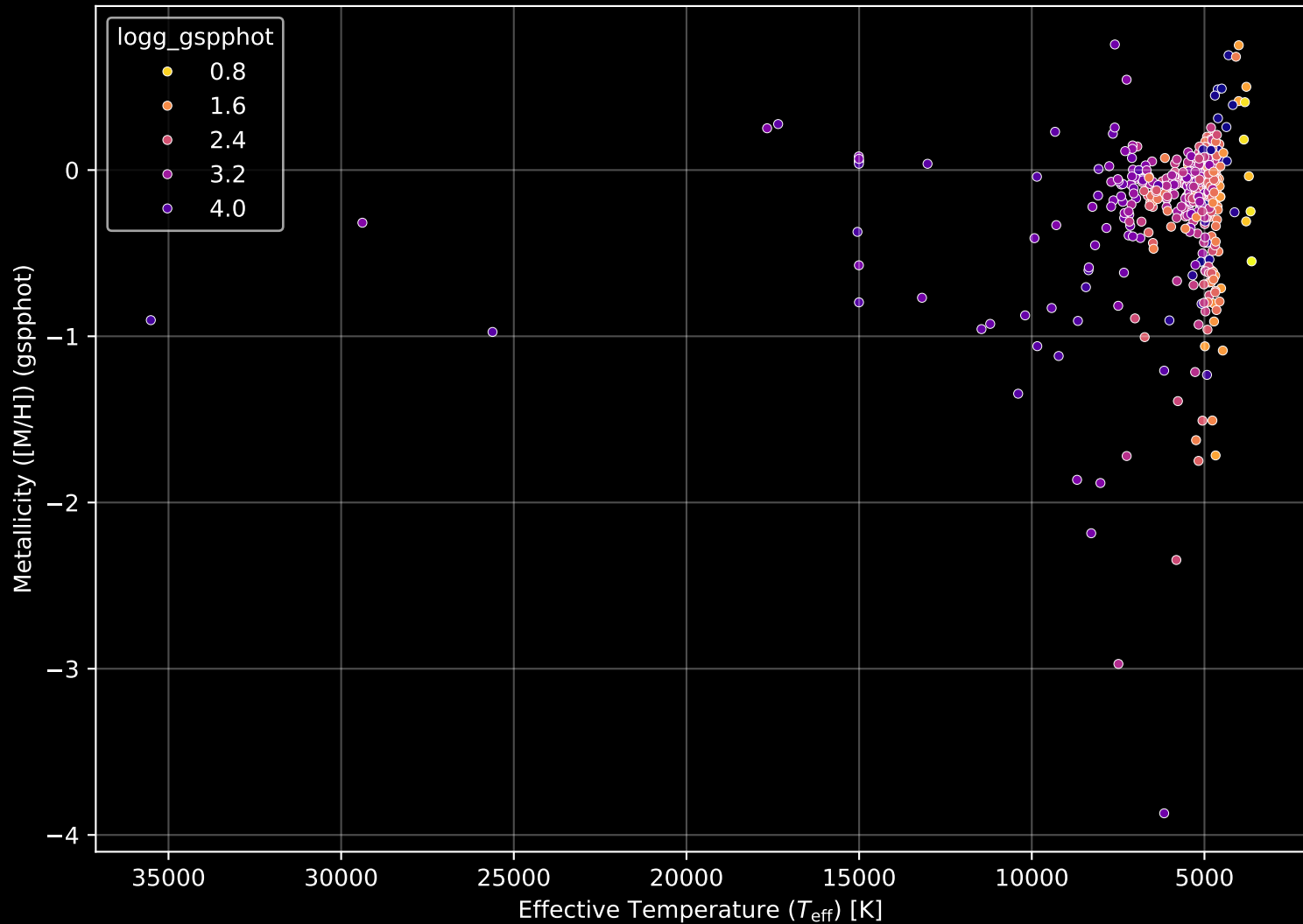
APOGEE DR17 Field: [184+00] Stellar Population Parameters (n= 440)
